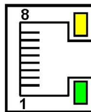
Rys. 37. Widok i numeracja pinów gniazda RJ45 miernika
