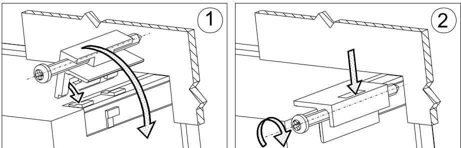
Rys. 2. Mocowanie miernika
