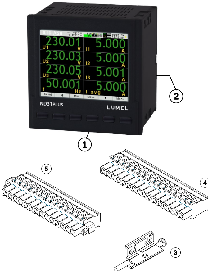
Rys. 1. Zestaw miernika
