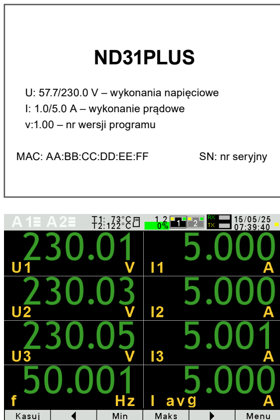
Rys. 11. Ekran trybu pomiarowego miernika
