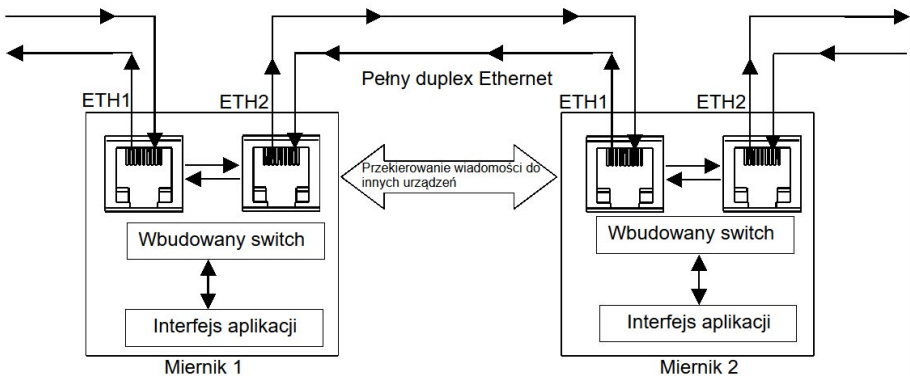
Rys. 36. Konfiguracja sieci Ethernet z 2-portowym switchem Ethernet
