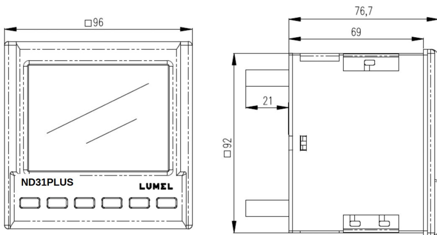
Rys. 3. Rysunek gabarytowy miernika ND31PLUS
